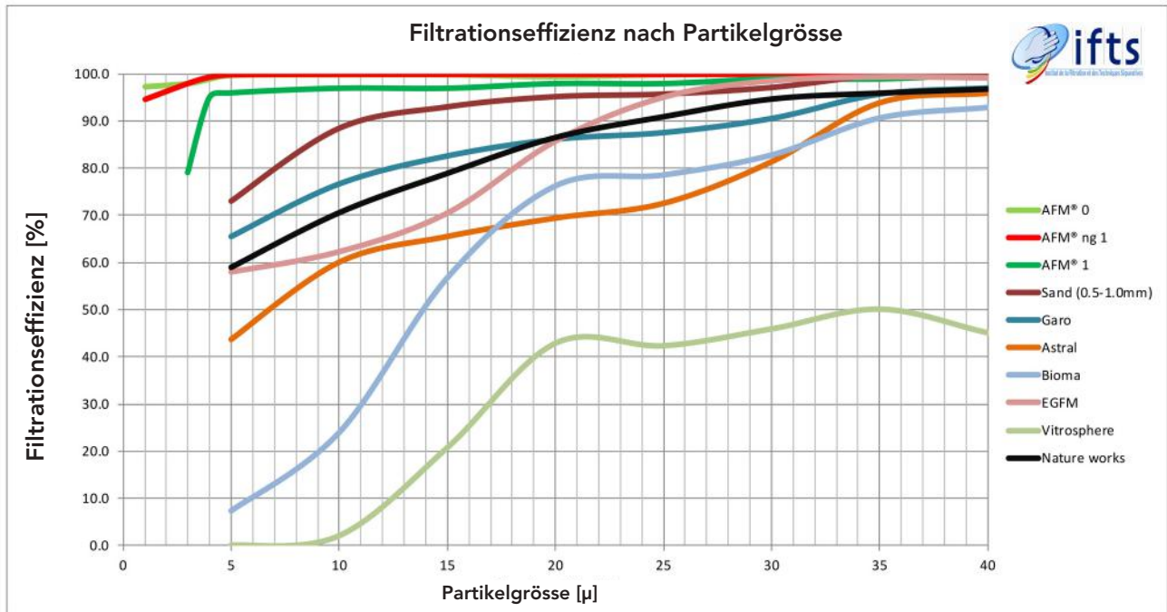
Grafik 1: Filtrationsleistung bei 20 m/h Filtrationsgeschwindigkeit und ohne Flockung.
